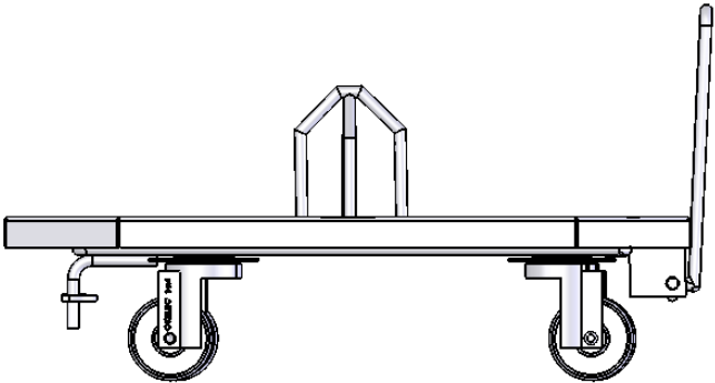
VUE GAUCHE
