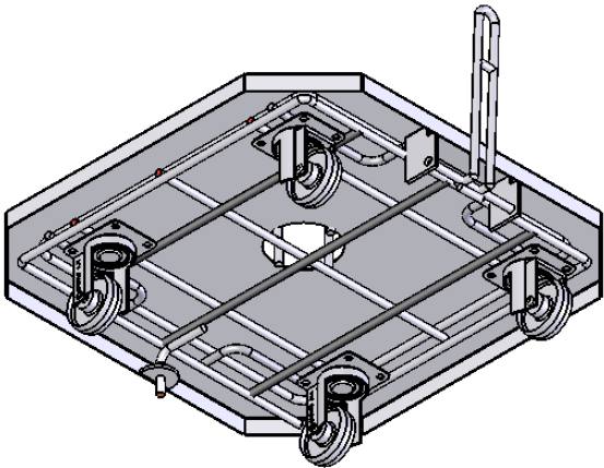
VUE 3D BAS
