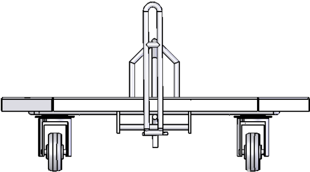
VUE AVANT
