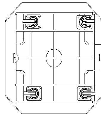
VUE DESOUS
